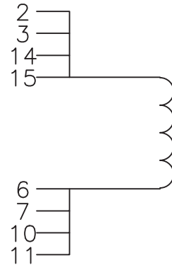
318 Schematic B
