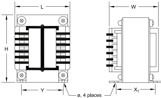
805-3, -4, -5 Side Views
