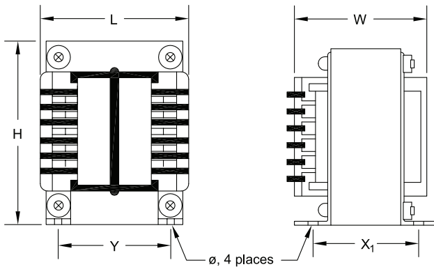
805-3, -4, -5 Side Views
