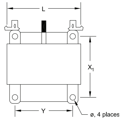
805-3, -4, -5 Top View
