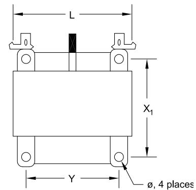
805-3, -4, -5 Top View
